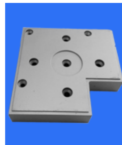
Picior EPC Culoare: ST* Dimensiune: 160mm
