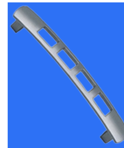
Mâner perforat pătrat Culoare: AL* Dimensiune: 96mm
